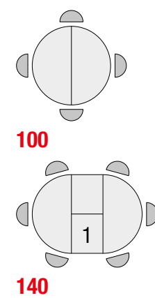
articolo 10018 Tavolo allungabile piano e allunga centrale da 40 cm. in gres porcellanato grigio chiaro opaco, meccanismo, gambe in acciaio antracite opaco. misura chiuso cm. l. 100 p. 100 h. 77 misura aperto cm. l. 140 p. 100 h. 75
